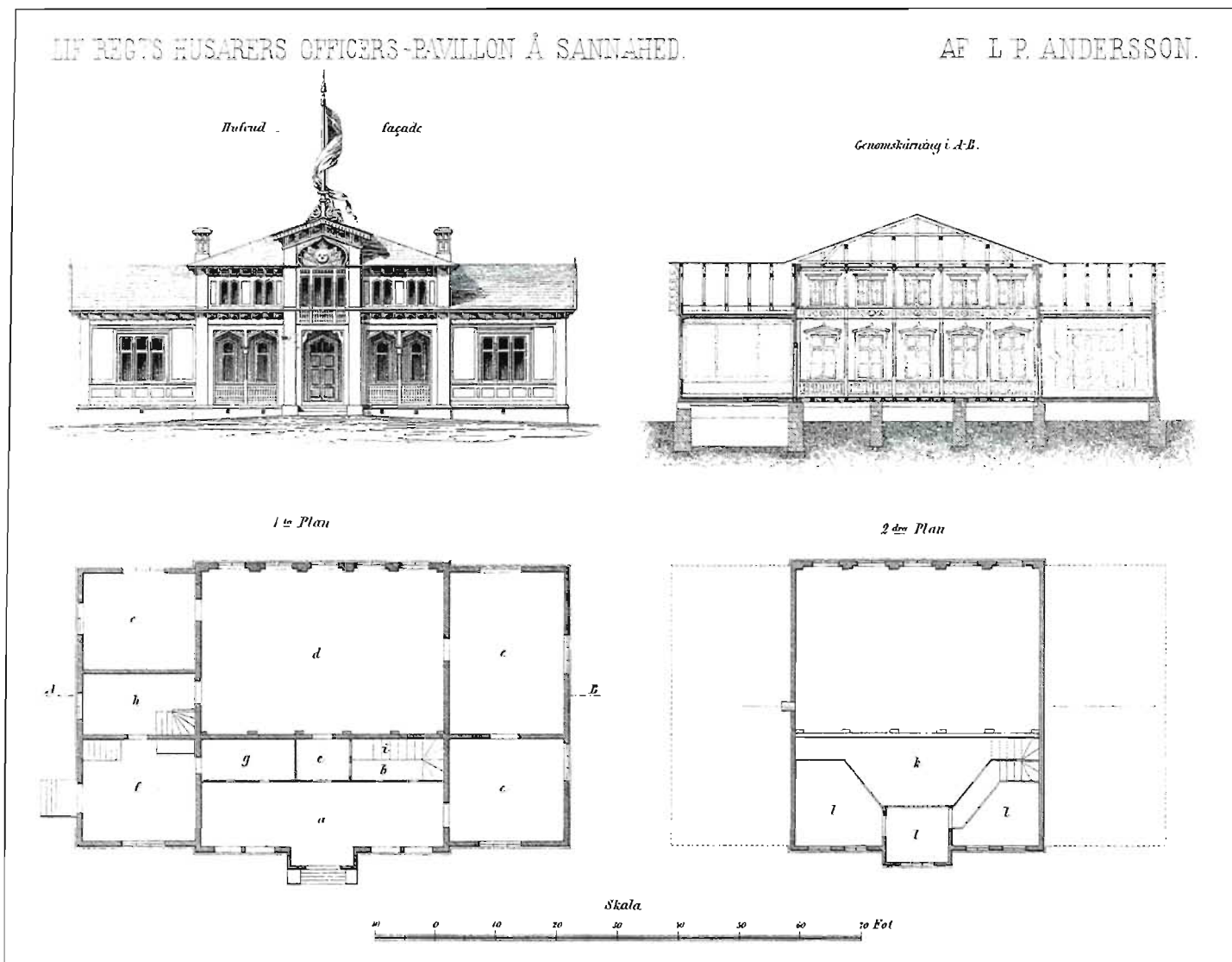
De av konduktören L. P. Andersson uppgjorda ritningarna till Livregementets husarers officersmäss i Sannahed. I texten finns förklaringar till de olika bokstavs-beteckningarna. Mässen stod vid husarläget — väster om Motorstadion — och uppfördes 1867 och flyttades 1909.
