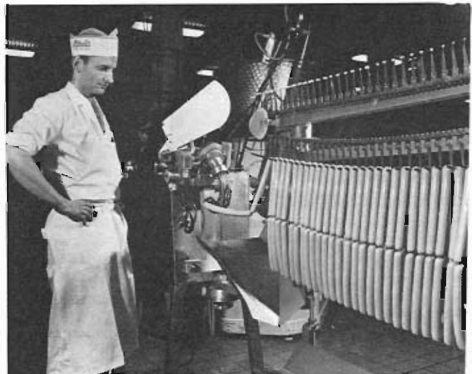
Den här moderna frank-a-matic-maskinen tar med hjälp av vacuum bort luften ur korvmassan, portionerar varje korv till exakt vikt, tvinnar av och hänger upp 300 korvar per minut.
