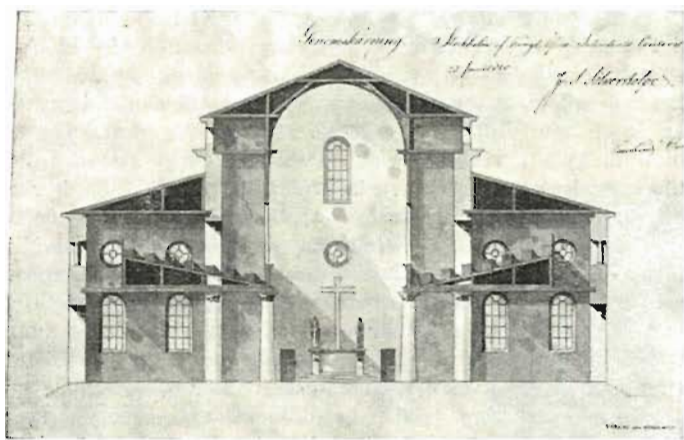
Bild 4. Genomskärning sedd mot koret Efter originalritning i Landsarkivet i Uppsala.
