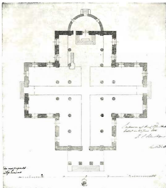
Bild 3. Planritning. Mörkare partier markera kvarblivande murverk från den gamla kyrkan.
