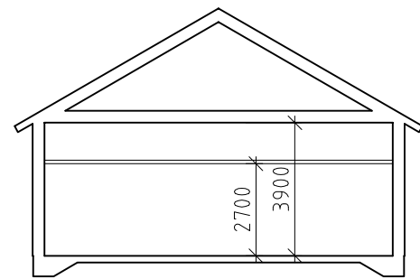
PRINCIPSEKTION A-A
